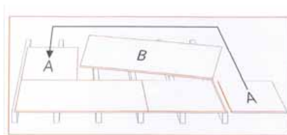
Plaatsen van houtvezelplaten Bron: Celit
