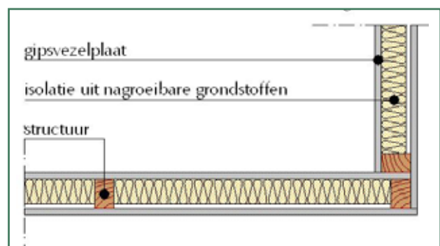
Aansluiting muur-muur, hoekverbinding Bron: Fermacell
